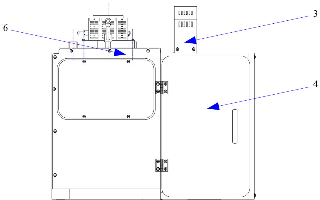
Zeichnung nr 16. Schematische Übersicht der Kessel Smart Fire SF 11 Compact und SF15 Compact: 1-Touch-Display; 2-Vorratsbehälter; 3-Abdeckung der Antriebseinheit der Förderschnecke; 4-Vorratsbehältersdeckel; 5-Abdeckung der Kesseltür; 6-Deckel der Revisionsöffnung am oberen Teil des Wärmetauschers;
