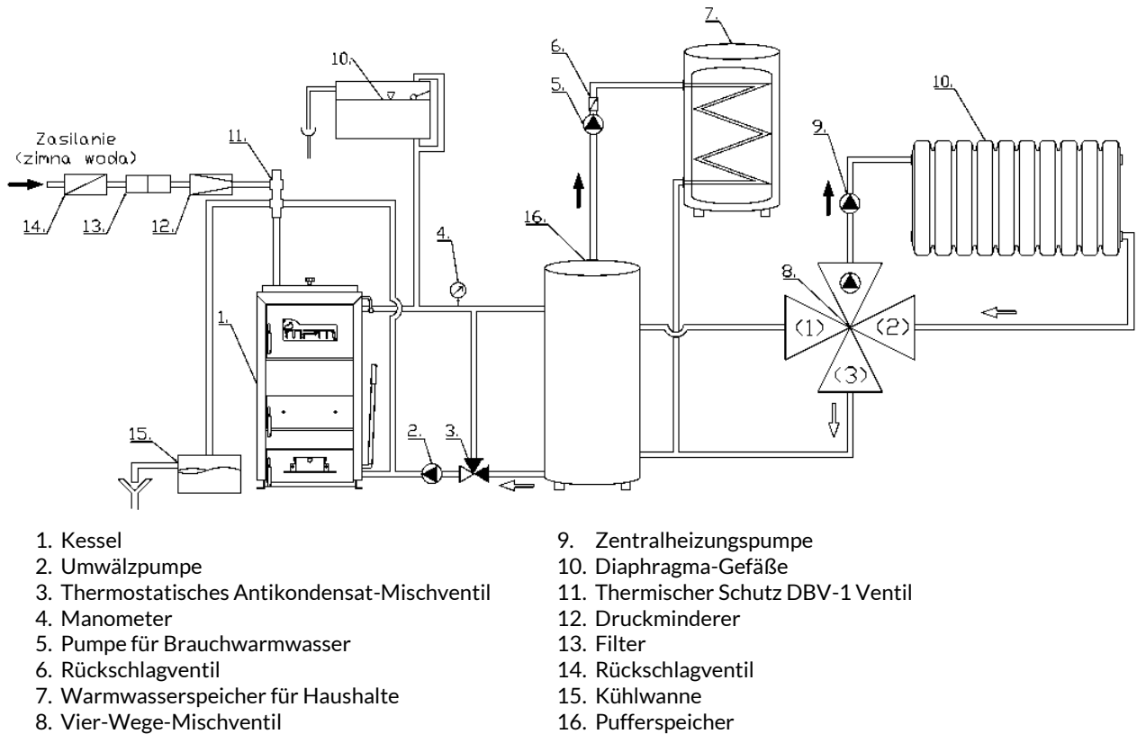
Abbildung 3: Beispielhafte Darstellung des Anschlusses des MPM Wood Plus Holzkessels in einem offenen System.
