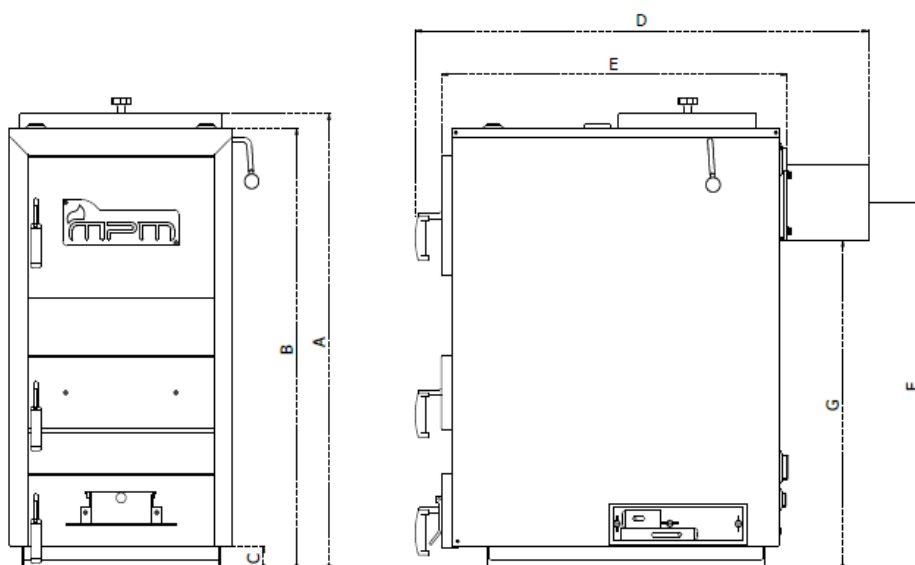
Abbildung 2: Grundlegende Abmessungen des MPM Wood Plus Holzkessels
