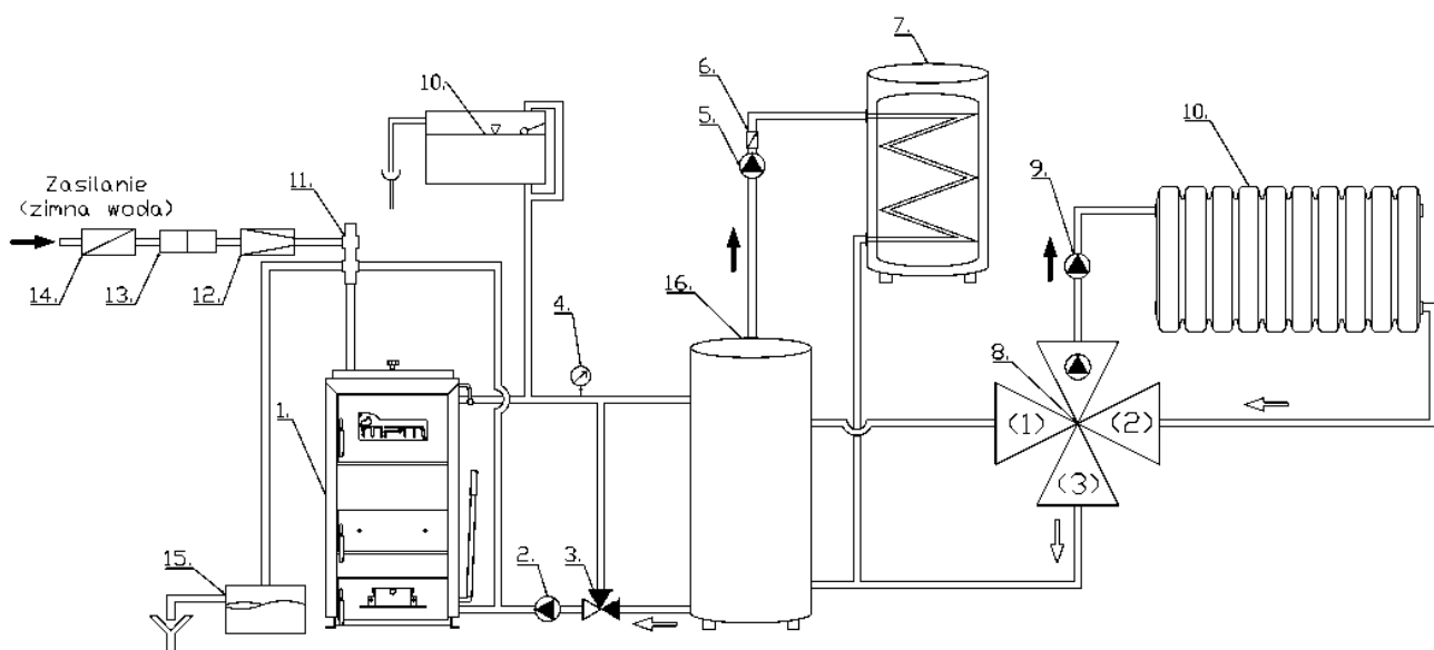
Abbildung 3: Beispielhafte Darstellung des Anschlusses des MPM Wood Plus Holzkeessels in einem offenen System.
