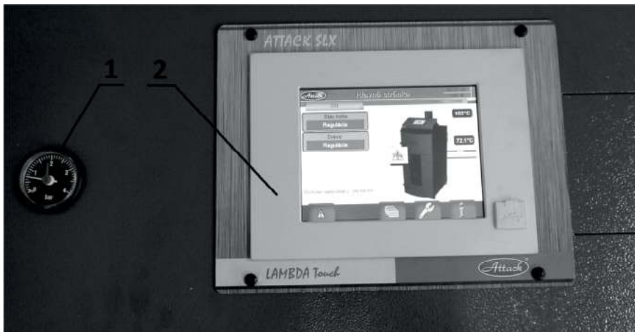
Bild 16. 1 – Manometer, 2 – Touchscreen
