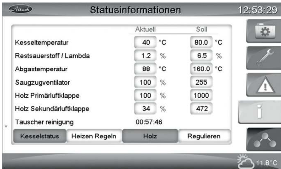
Bild 29. Regelregime
