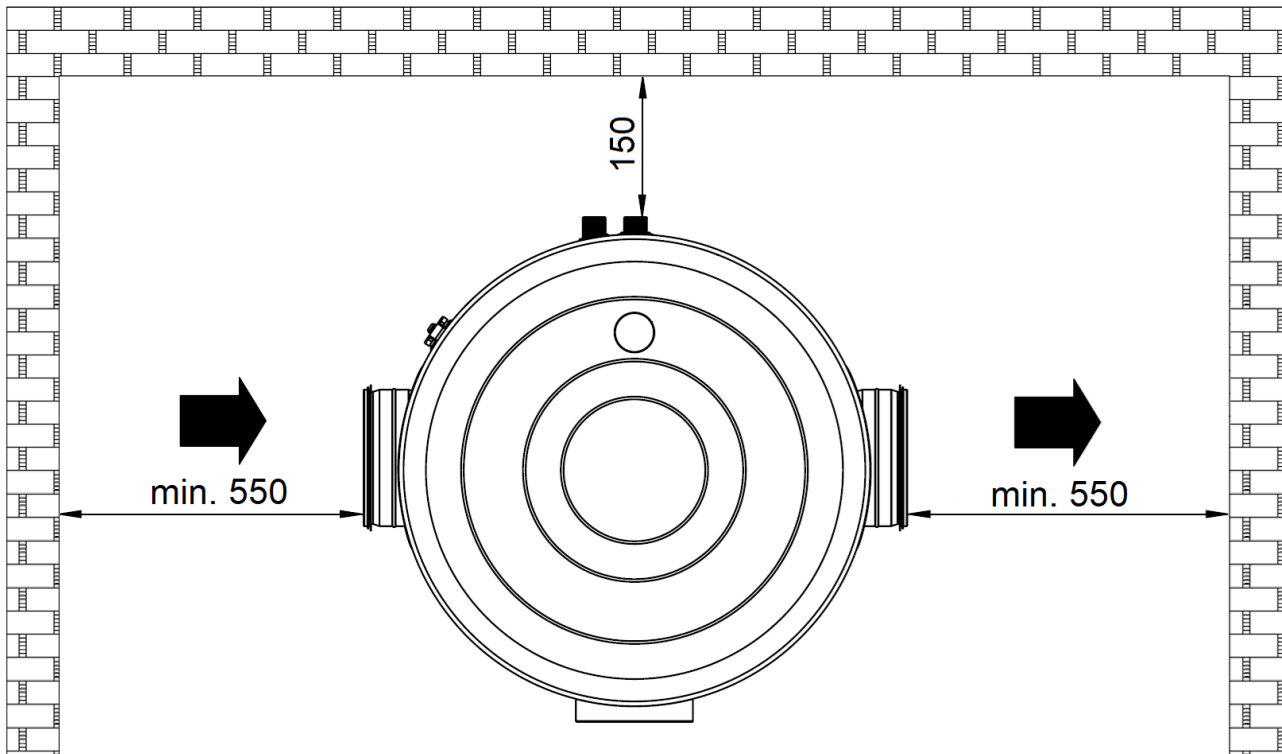
Abb. 4a. Installation der Wärmepumpe mit Einhaltung der erforderlichen Mindestabstände – Ansicht von oben.
