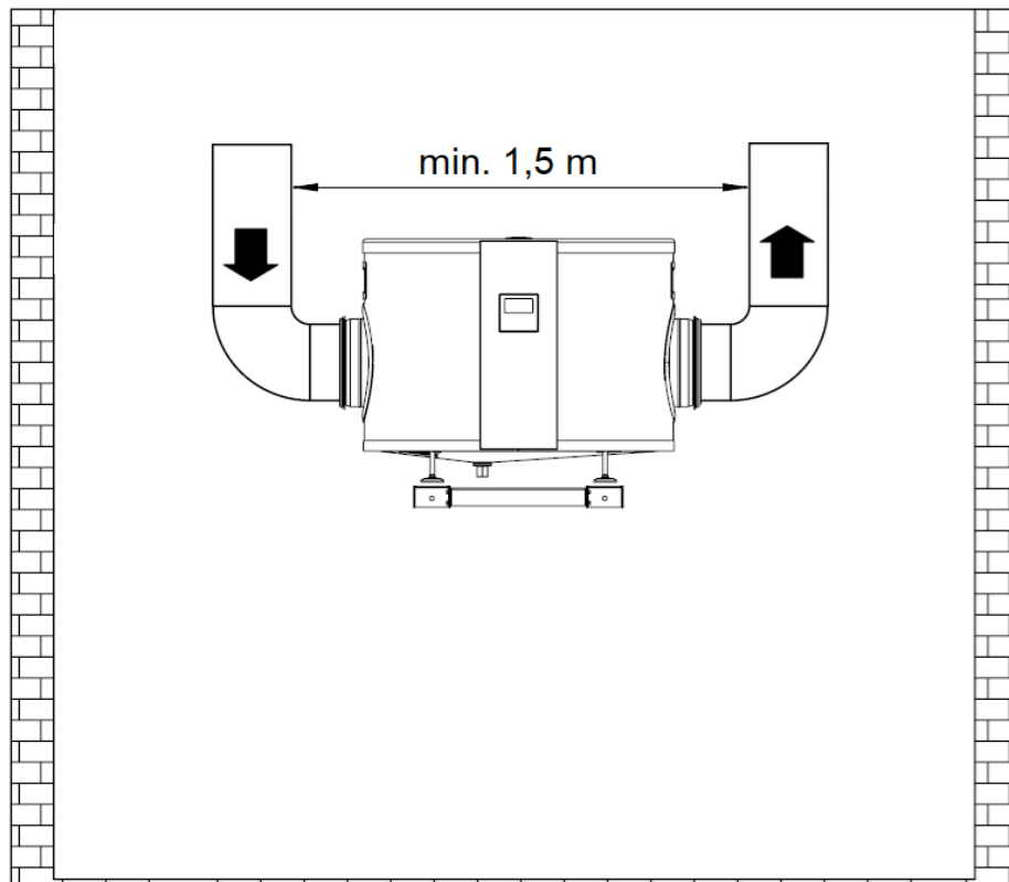
Abb. 7a. Mindestabstände zwischen den Luftkanälen – beispielhafte vertikale Montage.
