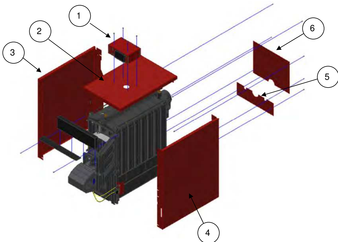
Abbildung 16 Verkleidungsmontage
